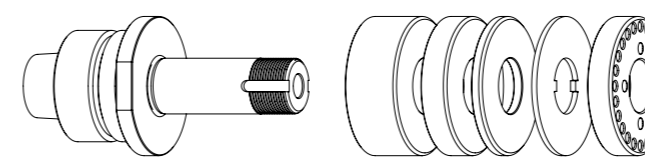
автоматика HSK-F40 // \varnothing 20 мм // Н. к. \varnothing 50 мм
