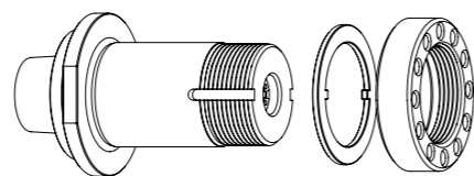
ручное управление HSK-F40 // \varnothing 32 мм // без Н. к.
