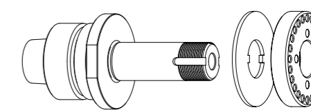
автоматика HSK-F40 // \varnothing 20 мм // без Н. к.
