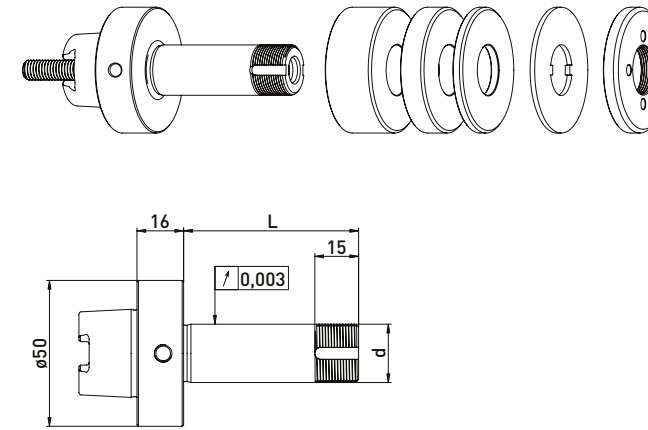
类似 HSK50 // \phi 20 毫米 // RS \phi 50 毫米
