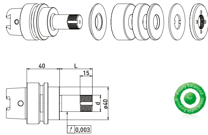
HSK50 // \phi 20 毫米 // RS \phi 50 毫米
