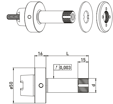
类似 HSK50 // \phi 20 毫米 // without RS
