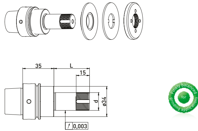
HSK-E40 // \phi 20 毫米 // without RS
