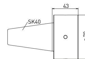
订购编号 名称 350130039 SK40转 Rollomatic 心轴25
