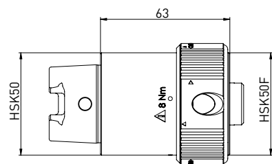
订购编号 名称 350130020 HSK50转 HSK40 A/C/E 与 HSK50 B/D/F
