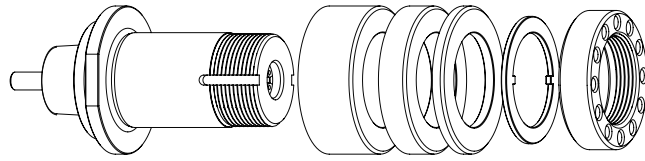
手动 HSK-F40 // \phi 32 毫米 // RS \phi 50 毫米
