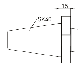
订购编号 名称 350130014 SK40转 Haas/Walter专用内锥
