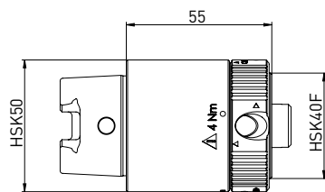
订购编号 名称 350130021 HSK50转 HSK32 A/C/E 与 HSK40 B/D/F
