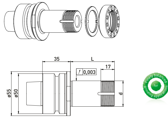
自动 HSK-F50 // \phi 32 毫米 // without RS
