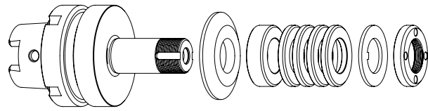
HSK50 NGC // \phi 20 毫米 // RS \phi 35 毫米
