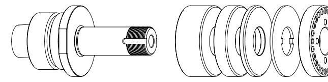
自动 HSK-F40 // \phi 20 毫米 // RS \phi 50 毫米
