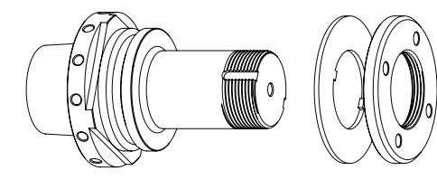
HSK-E50 // \phi 31,75 毫米 (1 1/4) // without RS
