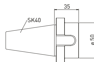
订购编号 名称 350130042 SK40转 Strausak内锥 (Promat)
