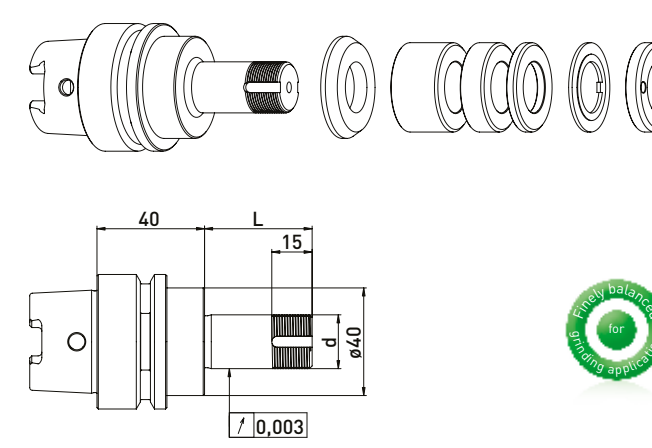
HSK50 // \phi 20 毫米 // RS \phi 35 毫米
