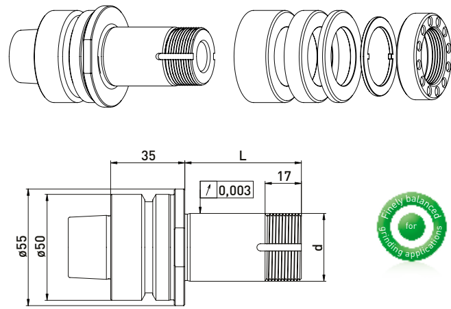
自动 HSK-F50 // \phi 32 毫米 // RS \phi 50 毫米
