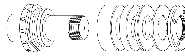
HSK-E50 // \phi 31,75 毫米 (1 1/4) // RS \phi 60 毫米
