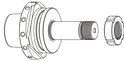
HSK-E50 // \phi 20 毫米 // without RS
