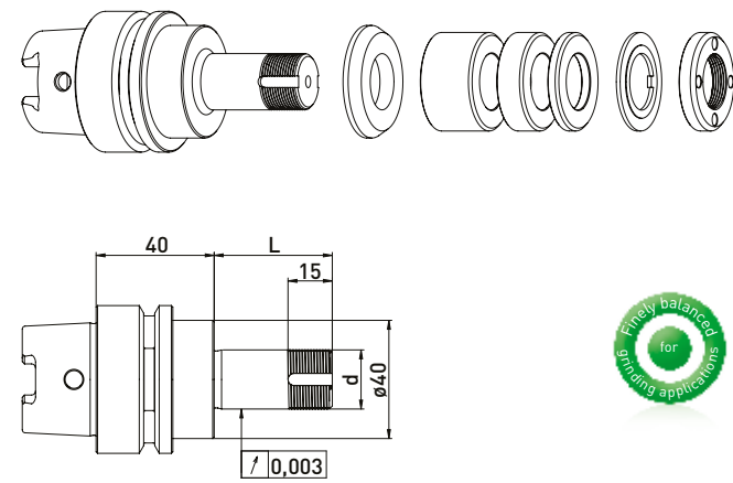
HSK50 // \phi 20 毫米 // RS \phi 35 毫米
