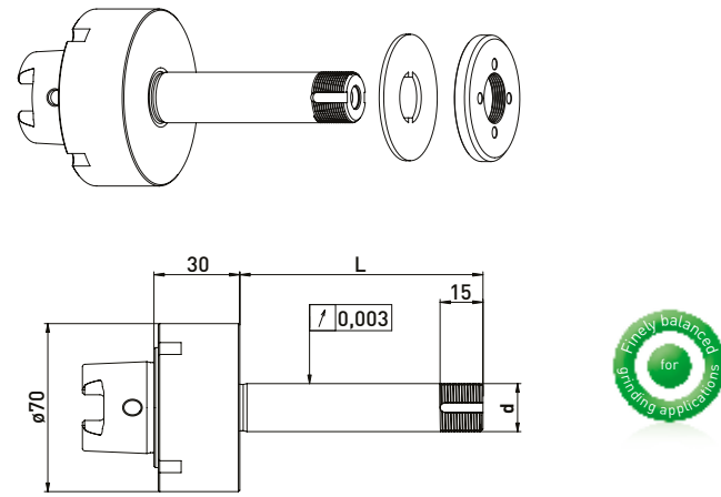
HSK50 // \phi 20 毫米 // without RS
