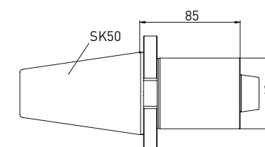
订购编号 名称 350130045 SK50转 Haas/Walter内锥 L85
