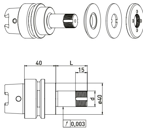
HSK50 // \phi 20 毫米 // without RS
