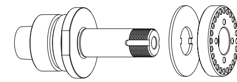
自动 HSK-F40 // \phi 20 毫米 // without RS
