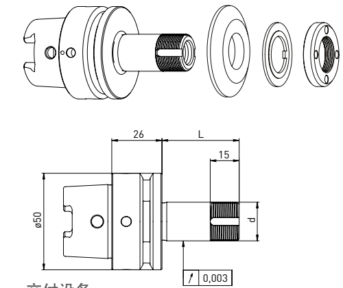
HSK50 // \phi 20 毫米 // without RS
