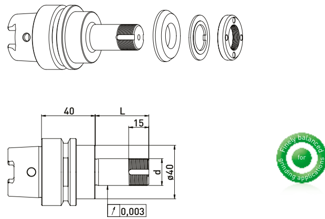
HSK50 // \phi 20 毫米 // without RS
