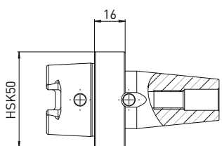
订购编号 名称 350130030 HSK50转 Strausak内锥 (Fleximat)
