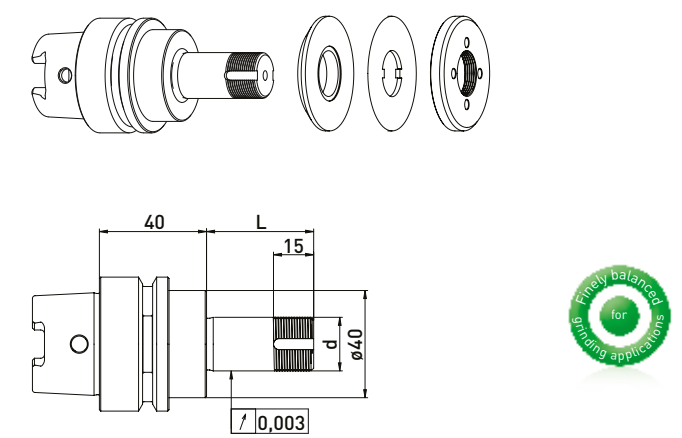
HSK50 // \phi 20 毫米 // without RS
