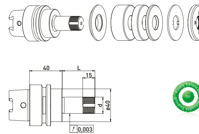
HSK50 // \phi 20 毫米 // RS \phi 50 毫米
