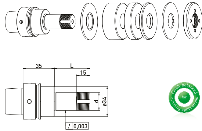
HSK-E40 // \phi 20 毫米 // RS \phi 50 毫米
