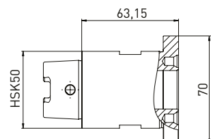
订购编号 名称 350130048 HSK50转 \times \phi 25 Rollomatic 心轴
