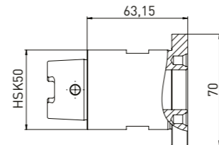
注文 No. 名称 350130048 アダプター (HSK50 x ø25を Rollomaticに接続)
