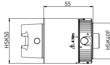
注文 No. 名称 350130021 アダプターピース (HSK50を HSK32 A/C/E HSK40 B/D/Fに接続)
