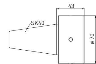
注文 No. 名称 350130039 アダプター (SK40を Rollomatic ø25に接続)
