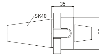
注文 No. 名称 350130035 アダプター (SK40を ANCAテーパーø30に接続)
