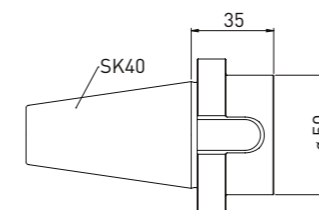
注文 No. 名称 350130042 アダプター (SK40を Strausak Promatに接続)
