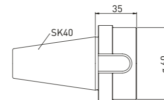
注文 No. 名称 350130040 アダプター (SK40を Saackeショートテーパーに接続)
