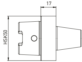
注文 No. 名称 350130034 アダプターピース (HSK50を ANCAテーパーø30に接続)
