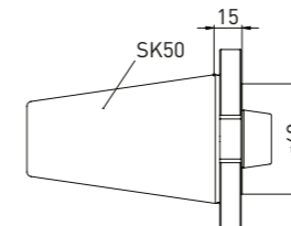
注文 No. 名称 350130044 アダプター (SK50を Haas/WalterテーパーL15に接続)
