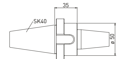
注文 No. 名称 350130043 アダプター (SK40を Strausak Fleximatに接続)
