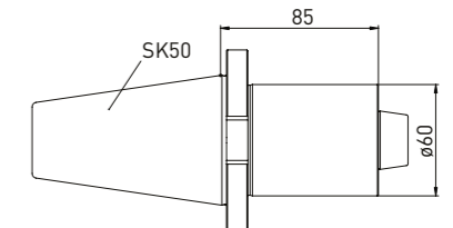
注文 No. 名称 350130045 アダプター (SK50を Haas/Walterテーパー L85に接続)
