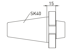
注文 No. 名称 350130014 アダプター (SK40を Haas/Walterテーパーに接続)
