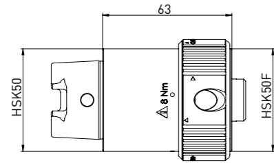
注文 No. 名称 350130020 アダプターピース (HSK50を HSK40 A/C/E HSK50 B/D/Fに接続)
