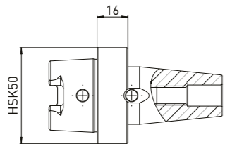
注文 No. 名称 350130030 アダプターピース (HSK50を Strausak Fleximatに接続)
