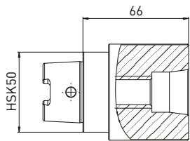
注文 No. 名称 350130033 アダプターピース (HSK50を Saackeショートテーパーに接続)
