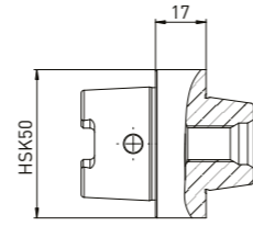
注文 No. 名称 350130032 アダプターピース (HSK50を Haas/Walterテーパーに接続)
