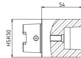
注文 No. 名称 350130031 アダプターピース (HSK50を Strausak Promatに接続)
