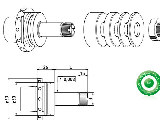
SSA HSK50E // \varnothing 20 mm // RS \varnothing 50 mm
