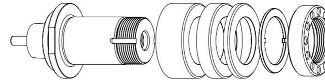
GWA manual HSK-F40 // \varnothing 31,75 mm (1¼) // RS \varnothing 50 mm
