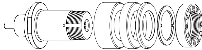
GWA manual HSK-F40 // \varnothing 32 mm // RS \varnothing 50 mm
