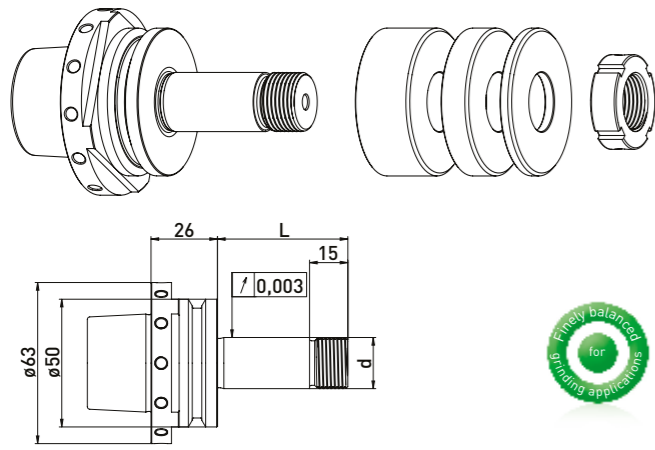
GWA HSK-E50 // \varnothing 20 mm // RS \varnothing 50 mm
