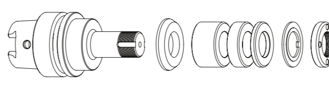
GWA HSK50 // \varnothing 20 mm // RS \varnothing 35 mm
