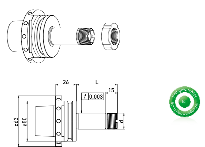
SSA HSK50E // \varnothing 20 mm // ohne RS
