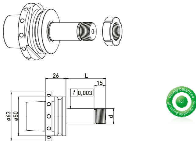
GWA HSK-E50 // \varnothing 20 mm // without RS
