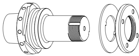
GWA HSK-E50 // \varnothing 31,75 mm (1¼) // without RS
