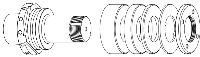
GWA HSK-E50 // \varnothing 31,75 mm (1¼) // RS \varnothing 60 mm
