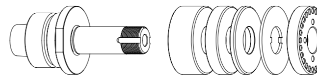
GWA manual HSK-F40 // \varnothing 20 mm // RS \varnothing 50 mm
